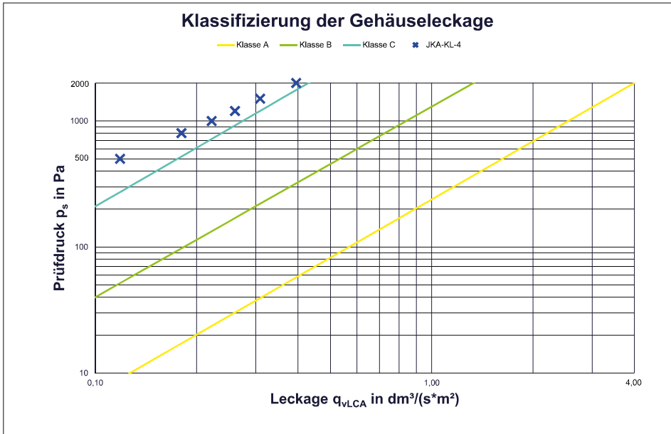
Abbildung 5: Gehäuseleckage „JKA-KL-4“
