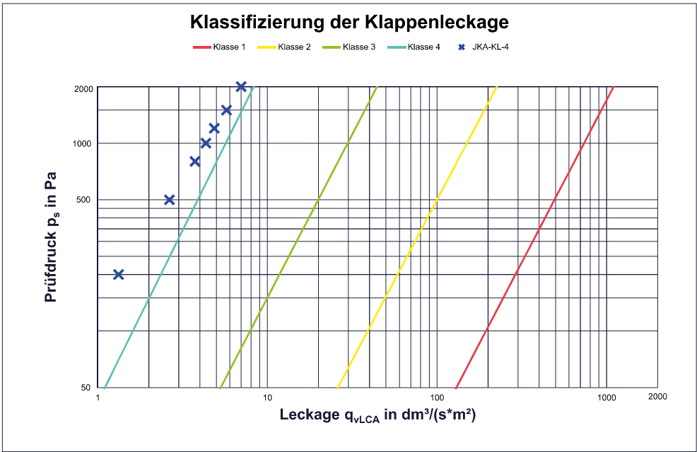
Abbildung 6: Klappenleckage „JKA-KL-4“
